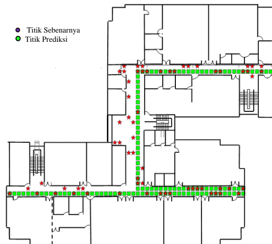
Gambar 10. Hasil prediksi metode NB untuk luasan 2\text{ m}^2
